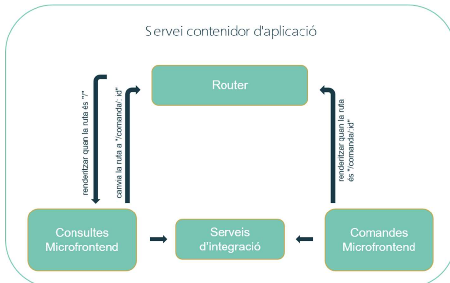
Il·lustració 25 Servei contenidor d'aplicació amb serveis d'integració
