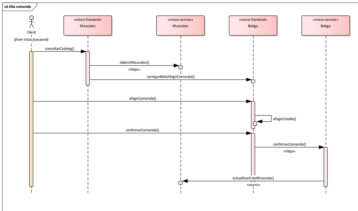
Il·lustració 5 Diagrama de seqüència
