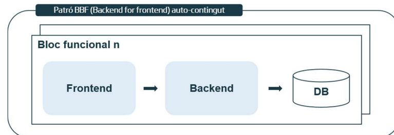
Il·lustració 7 Patró Backend for frontend
