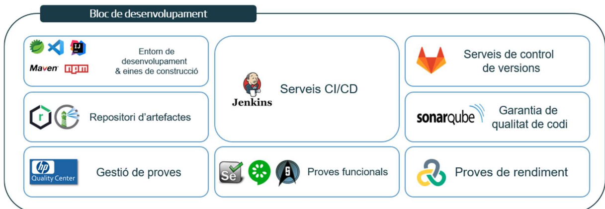
Il·lustració 27 Disseny lògic. Arquitectura de desenvolupament
