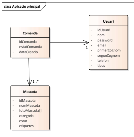
II-lustració 6 Diagrama global PetStore
