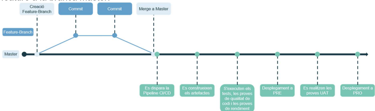
Il·lustració 10 Branching
