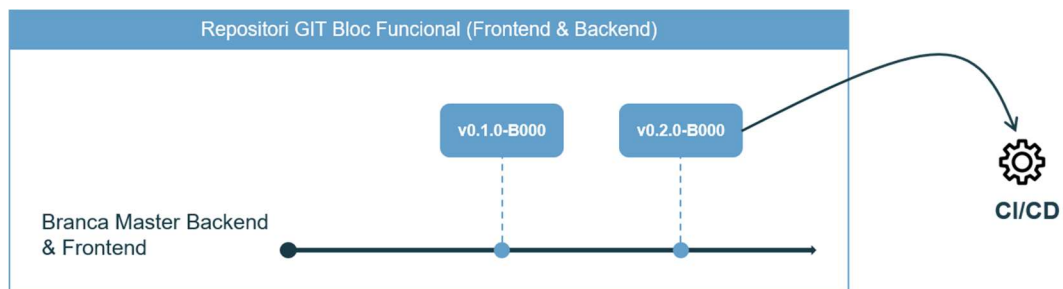
II-lustració 9 Versionat
