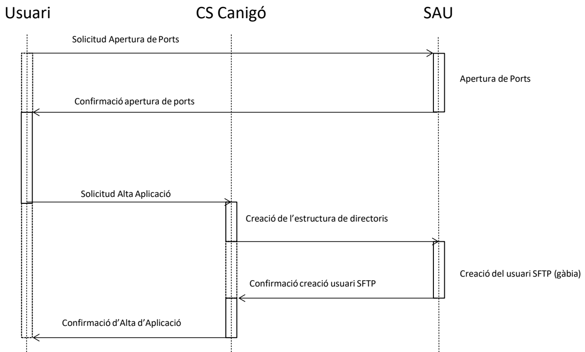
Figura 2.4 – 1. Esquema de peticions
