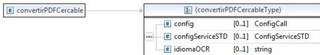
Taula 4.4.4 – 1. Camps d'entrada del servei convertirPDFCercable
